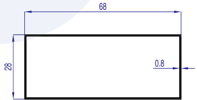
AU 7990 WEIGHT 0.380 Kg/m
