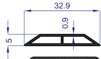
AU 71937 WEIGHT 0.164 Kg/m
