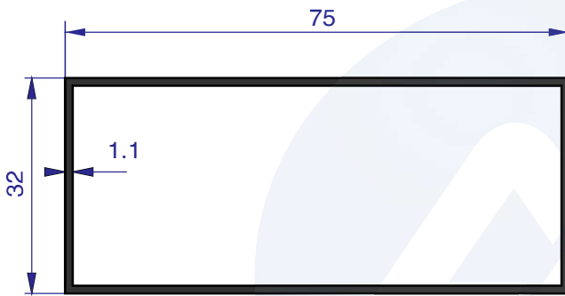
AU 7998 WEIGHT 0.625 Kg/m
