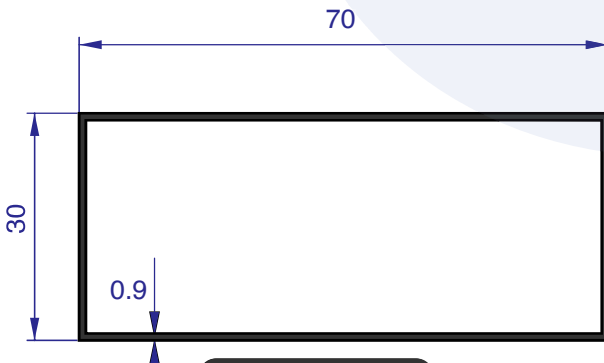
AU 71001 WEIGHT 0.479 Kg/m
