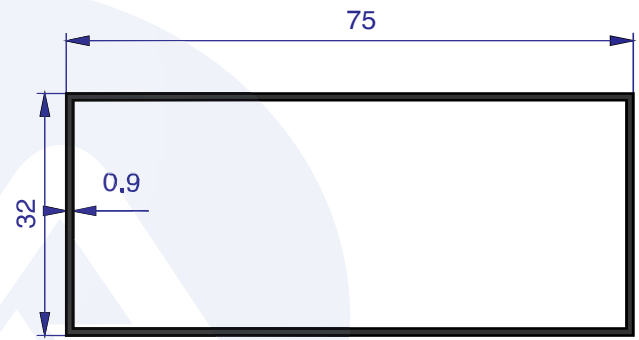
AU 7991 WEIGHT 0.363 Kg/m
