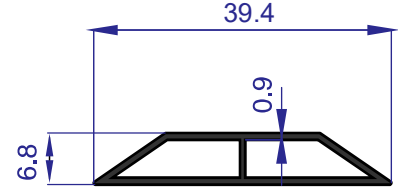
AU 71938 WEIGHT 0.191 Kg/m
