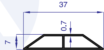
AU 7992 WEIGHT 0.155 Kg/m
