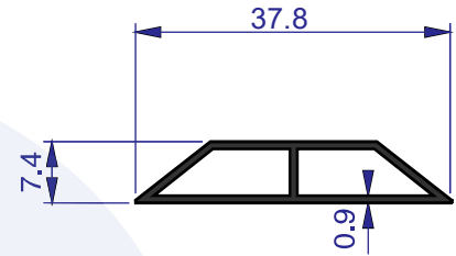
AU 7997 WEIGHT 0.201 Kg/m
