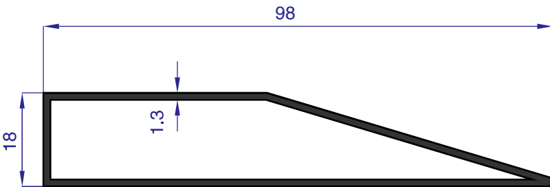
AU 72270 WEIGHT 0.775 Kg/m
