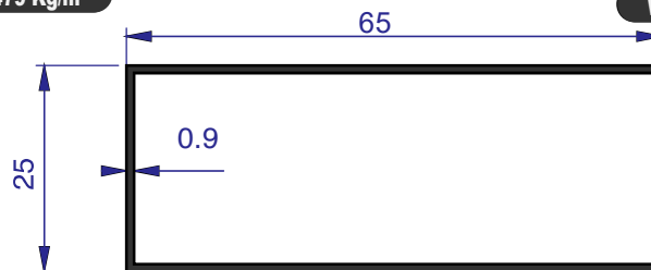
AU 71000 WEIGHT 0.430 Kg/m
