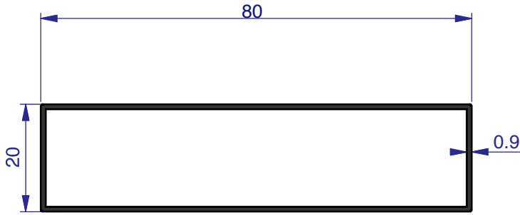
AU 7996 WEIGHT 0.478 Kg/m
