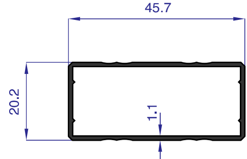
AU 7991 WEIGHT 0.363 Kg/m
