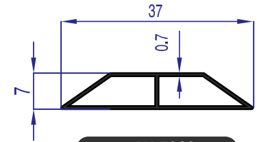
AU 7989 WEIGHT 0.144 Kg/m
